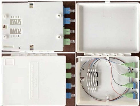
ODF 04 ( Size: H: 140, W: 116, D: 30mm)
