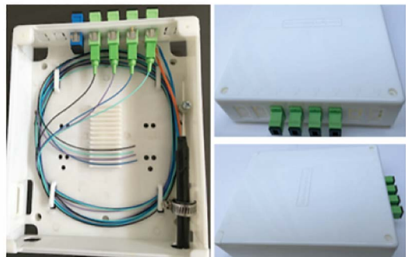
ODF 08 ( Size: H: 170, W: 140, D: 38mm)
